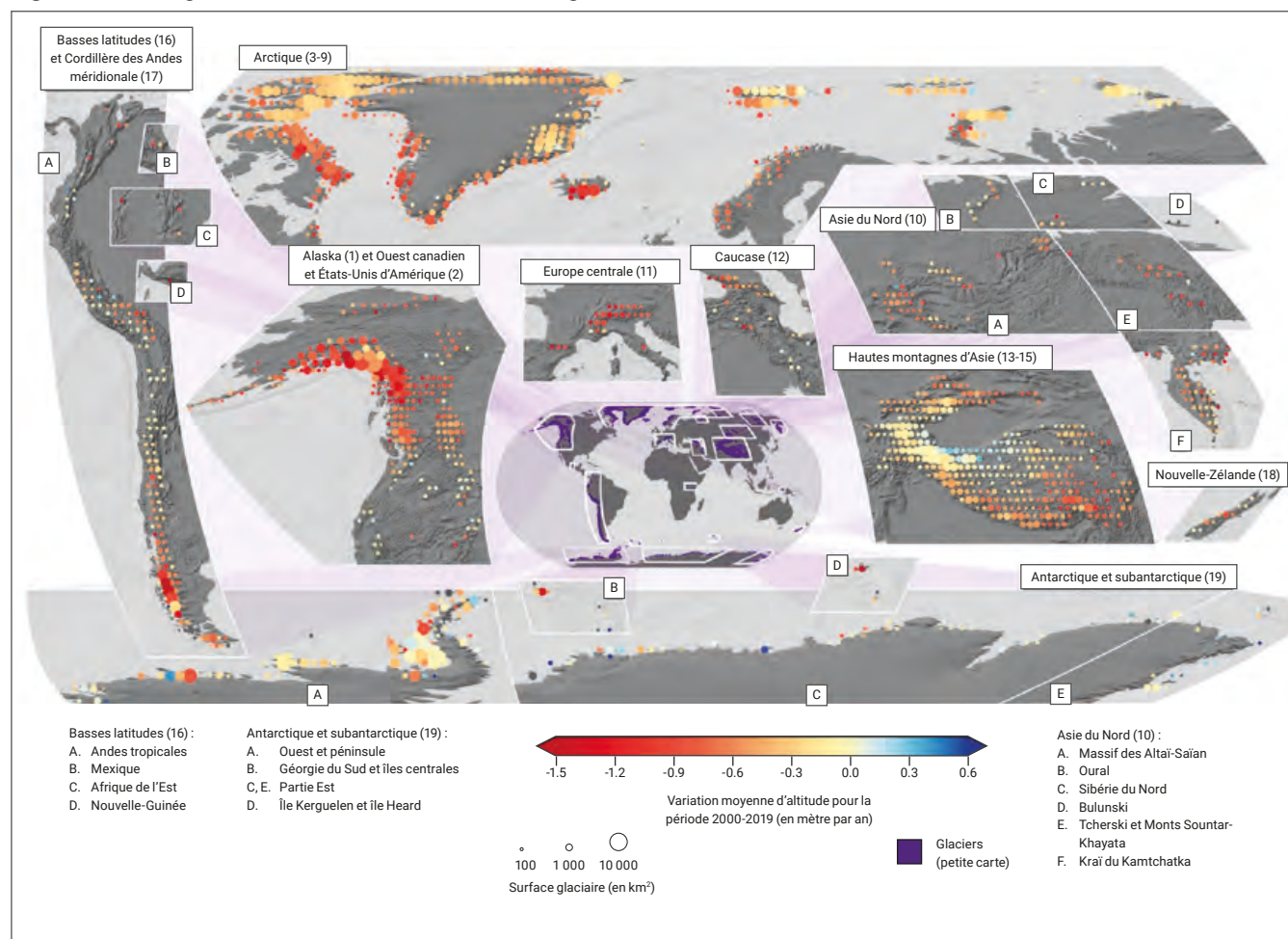
Figure 2.4 Changements d'altitude de la surface des glaciers dans le monde, 2000-2019
