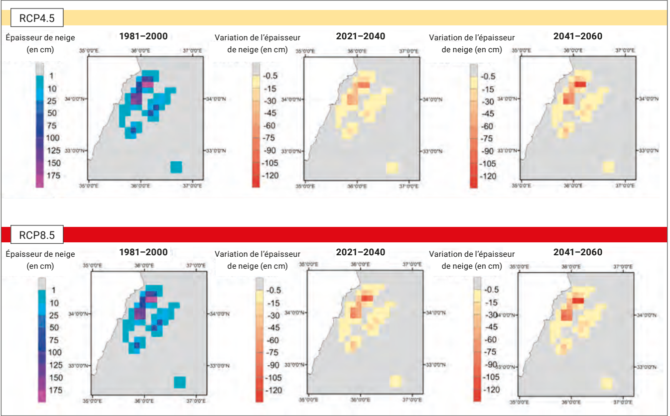
Figure 7.11 Évolution de l'épaisseur moyenne saisonnière de la neige (octobre à mars) sur le mont Liban pour les périodes 1981-2000, 2021-2040 et 2041-2060
