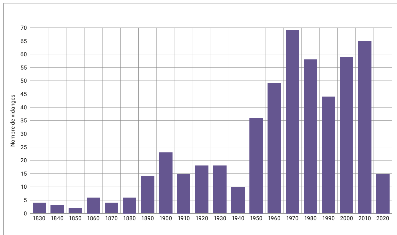
Figure 7.6 Nombre de vidanges brutales de lacs glaciaires enregistrées par décennie dans les régions de haute montagne d'Asie, décennies de 1830 à 2020
